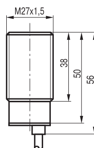
Габаритный чертеж
